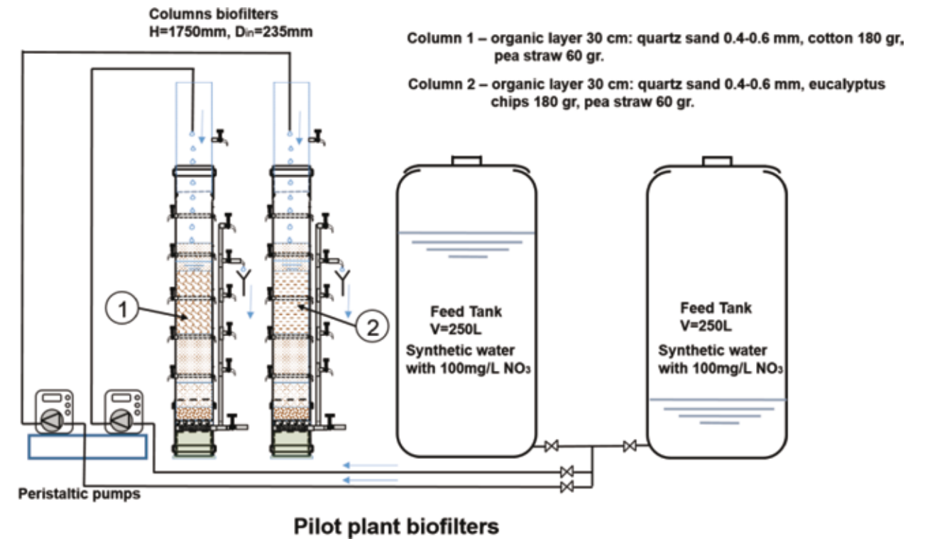
איור 30: תמונת מערכת הפילוט עם שתי קולונות דניטריפיקציה במצעי כותנה/קש ושבבי עץ/קש
