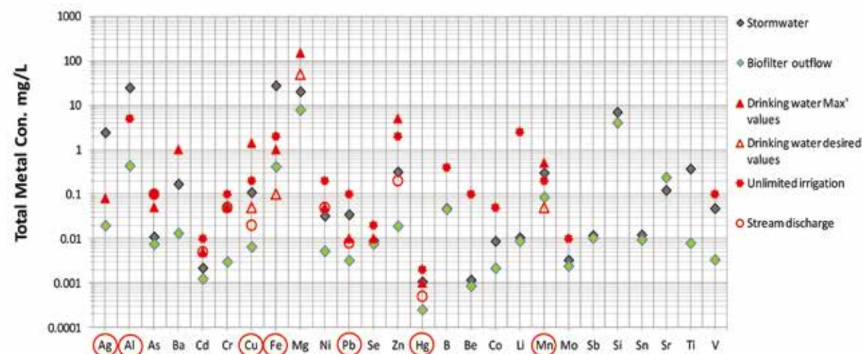
איור 44: ריכוזים ממוצעים של מזהמים לאירוע גשם עבור מתכות כבדות בכניסה לביופילטר (באפור) ומי נגר מטהרים ביציאה מהביופילטר (בירוק) בהשוואה לתקני איכות מים שונים (באדום)
