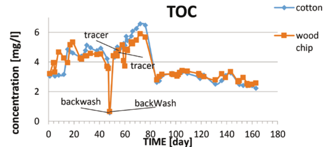
איור 35: ערכי TOC ביציאה מקולונות הכותנה ושבבי העץ לאורך הזמן
