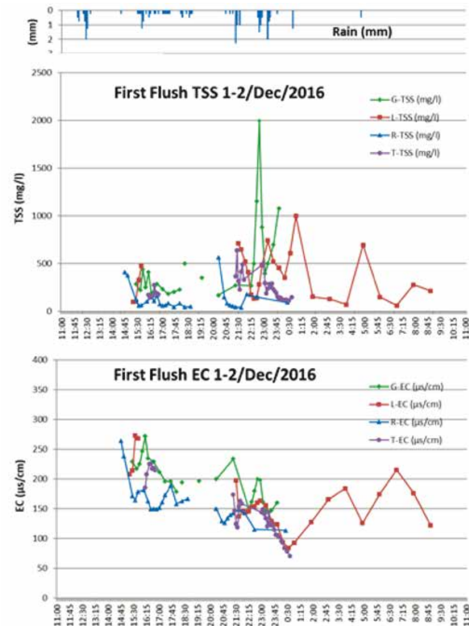
איור 15: TSS, EC כולטוגרף של הגשם הראשון ב-1-2 לדצמבר 2016
