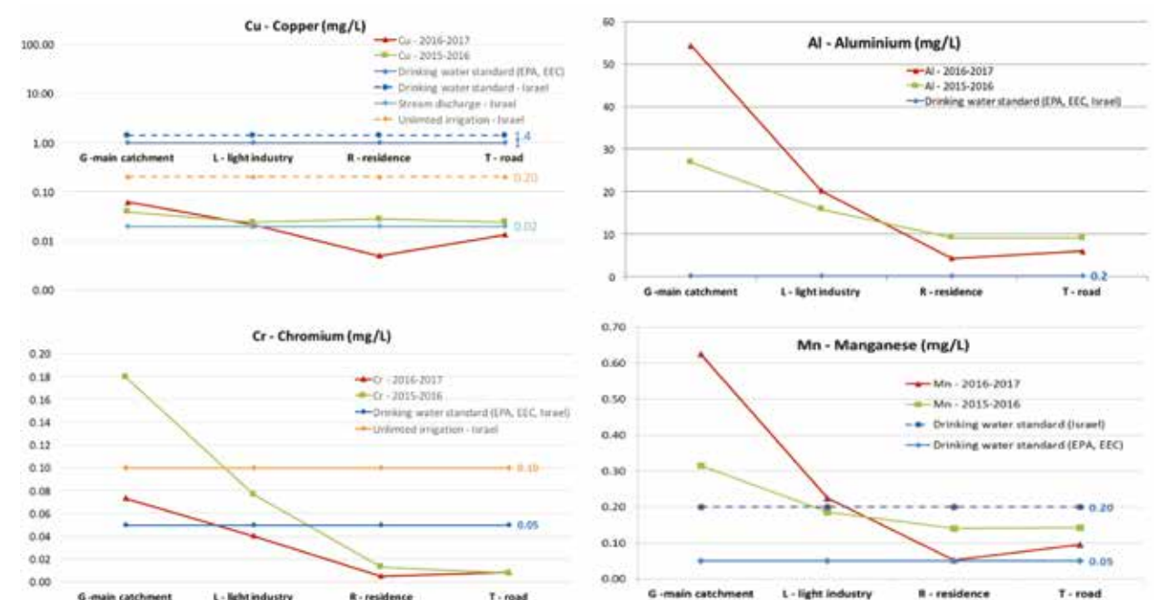
איור 18: השוואת ריכוזים עונתיים של Cu, Cr, Al, לתקני המים השונים
