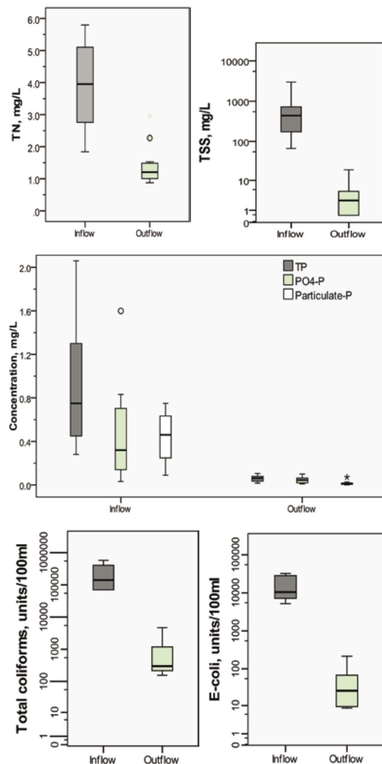
איור 42: ריכוזים ממוצעים לאירועי גשם-נגר בכניסה (מי נגר גולמיים - לפני טיפול בצבע אפור) וביציאה מהביופילטר (מי נגר מטוהרים - לאחר טיפול בצבע ירוק)
