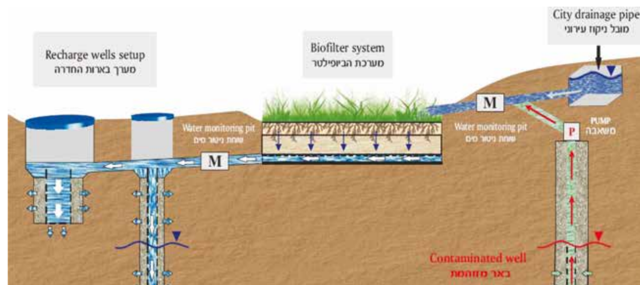
איור 41: מערכת הביופילטר ההיברידי בכפר-סבא מציגה עקרון פעולה דו שימושי ורב עונתי (קצירת מי נגר בחורף וידיאליזת אקוויפר בקיץ).
