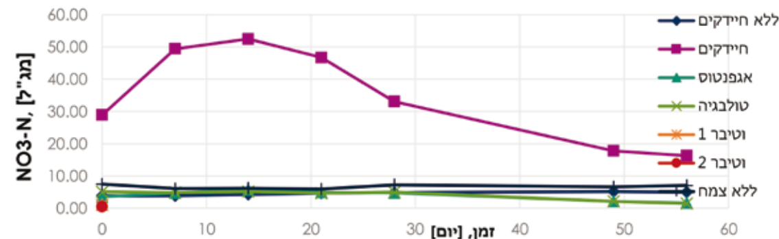
איור 37: ערכי ניטרט ביציאה מהקולונות בתפעול להדמיית טיפול במי-שיטפונות
