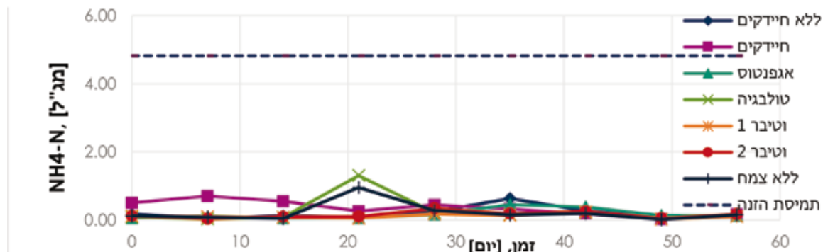
איור 36: ערכי אמוניה ביציאה מהקולונות בתפעול להדמיית טיפול במי-שיטפונות
